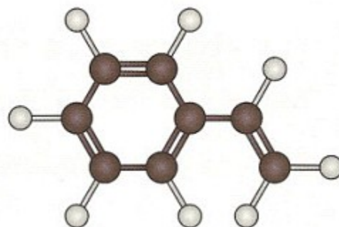
styrène
