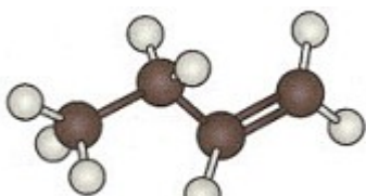
but-1-ène
