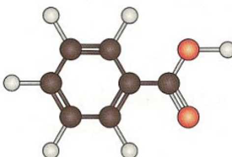
Acide benzoïque
