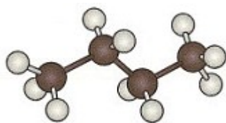
butane
