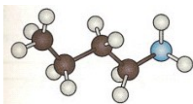
butan-1-amine
