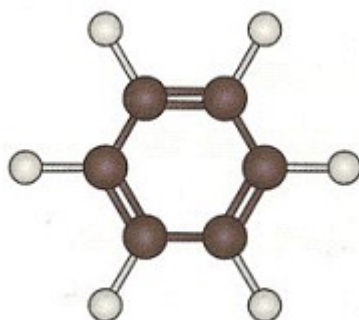
benzène
